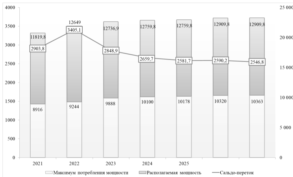
Рисунок 7.1. Баланс мощности по энергосистеме Иркутской области в период 2022-2027 гг. для дополнительного варианта развития (МВт)
