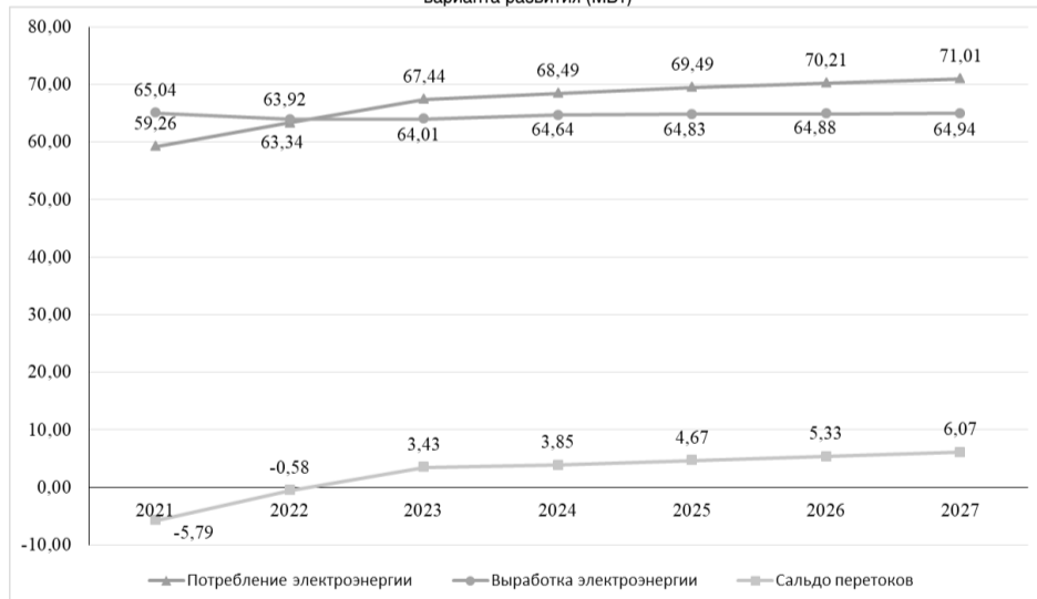
Рисунок 7.2. Баланс электроэнергии по энергосистеме Иркутской области в период 2022-2027 гг. для дополнительного варианта развития (млрд кВт*ч)
