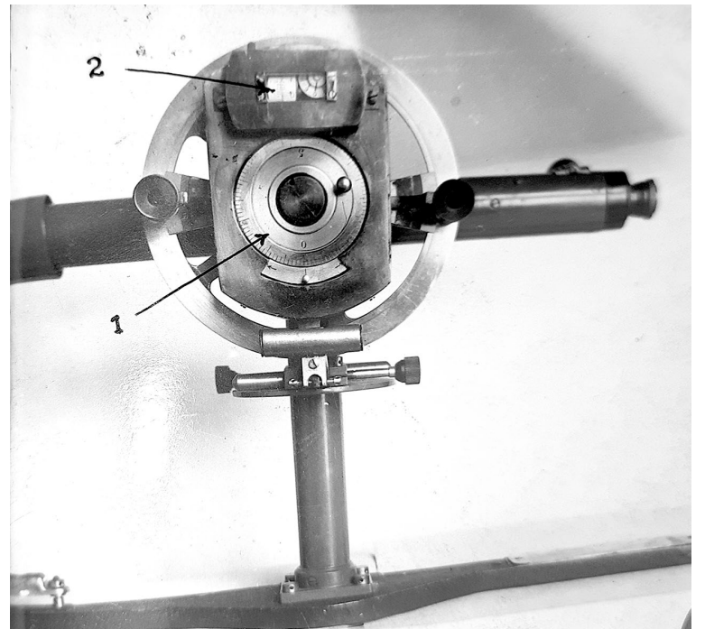
Высотомер инженера Григория Стодолкевича
