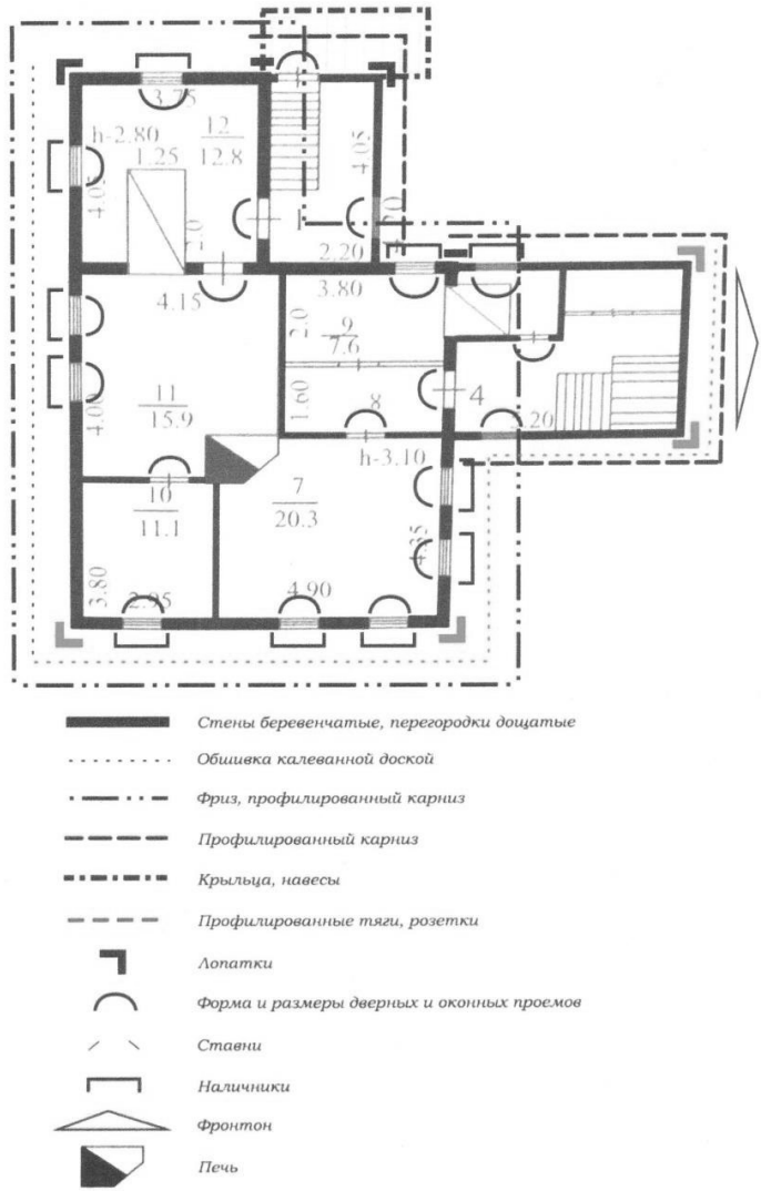
Дом лит Л. Схема расположения предмета охраны (ценных элементов) второго этажа
