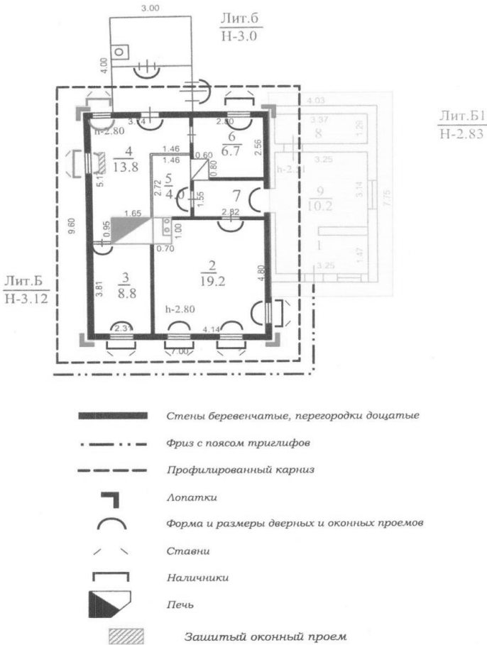
Дом лит Б. Схема расположения предмета охраны (ценных элементов) первого этажа
