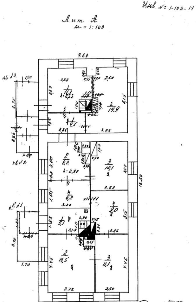
м.р. 12.1.83г. м.с. Курякова м.р. 2/1-80г. Байкальска Заснято: 18.07.84г. Тек. рез. 1.11.84г. С.М. Мамеж Рис.2 - Поэтажный план 1983г.
