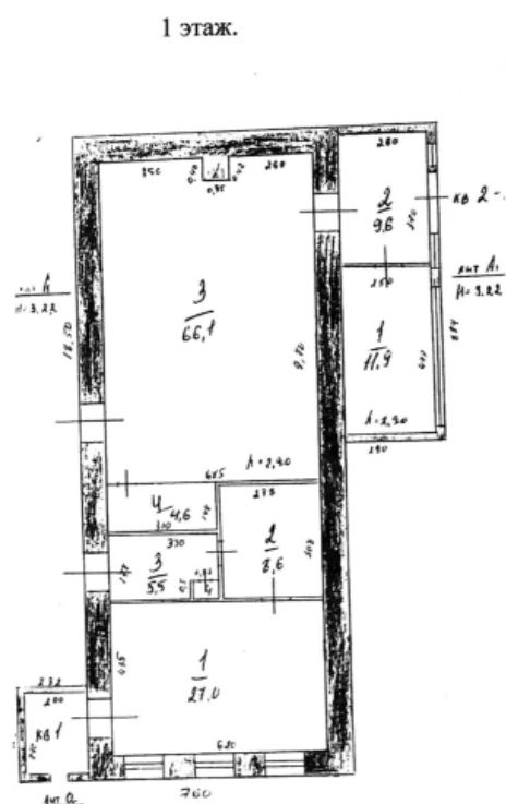
Рис.4 - поэтажный план 2001г.
