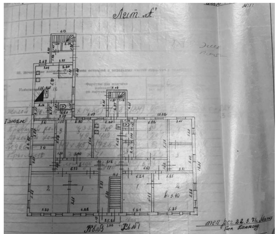
Рис. 4. План БТИ
