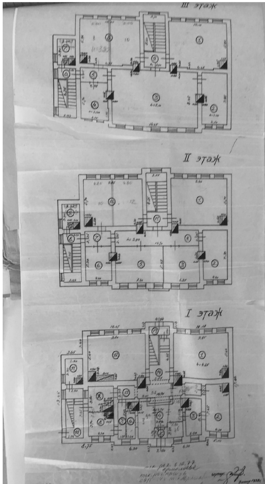
Поэтажные планы здания лит. А. Инвентаризация БТИ 1934 – 1977 г.
