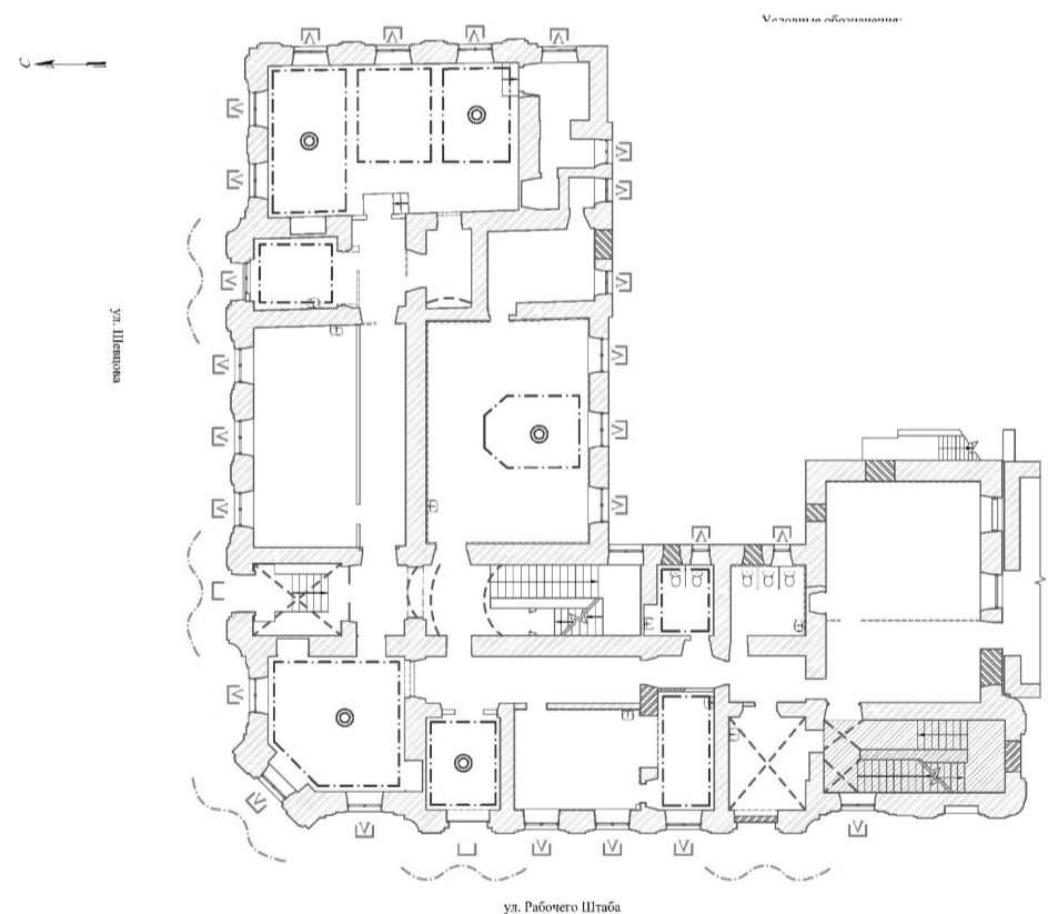
Схема размещения особенностей объекта культурного наследия (предмета охраны). План 1-го этажа
