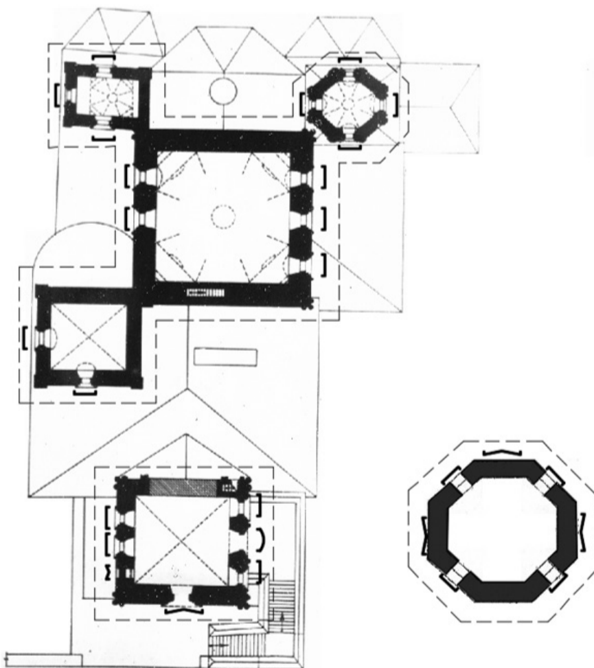
Схема расположения предмета охраны (ценных элементов) второго и третьего этажей Собора Богоявления
