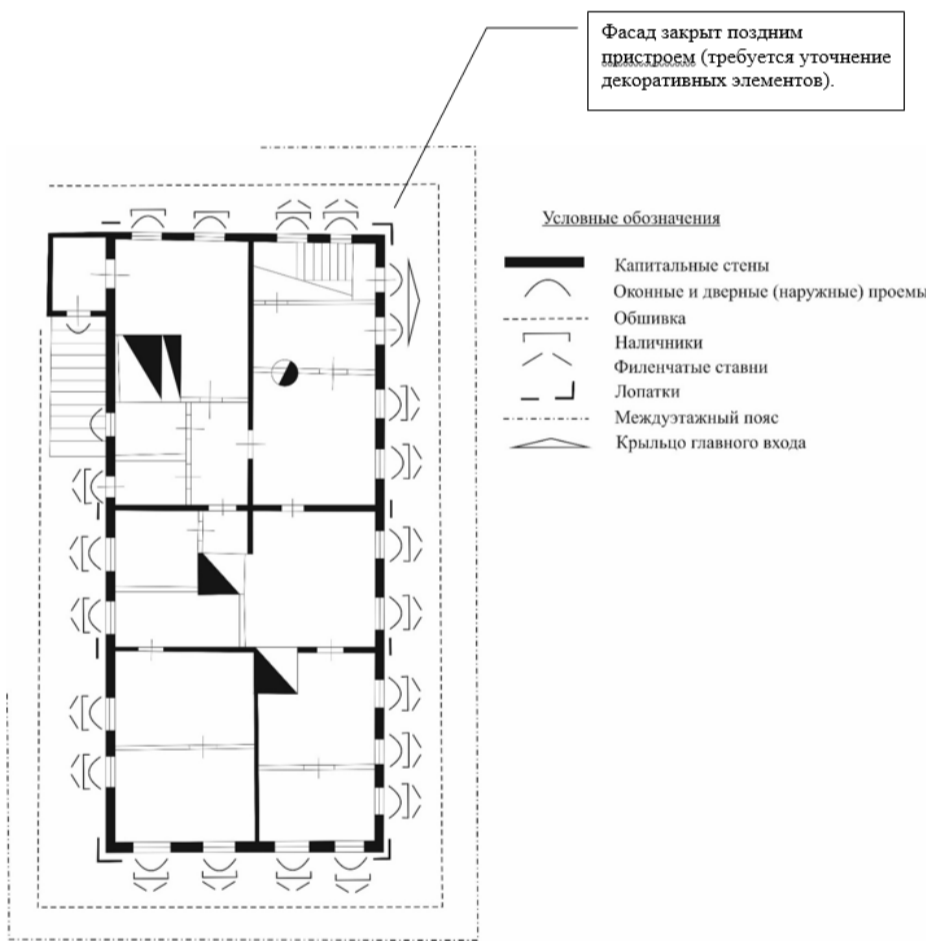
Схема обозначения предметов охраны объекта культурного наследия 1 этаж
