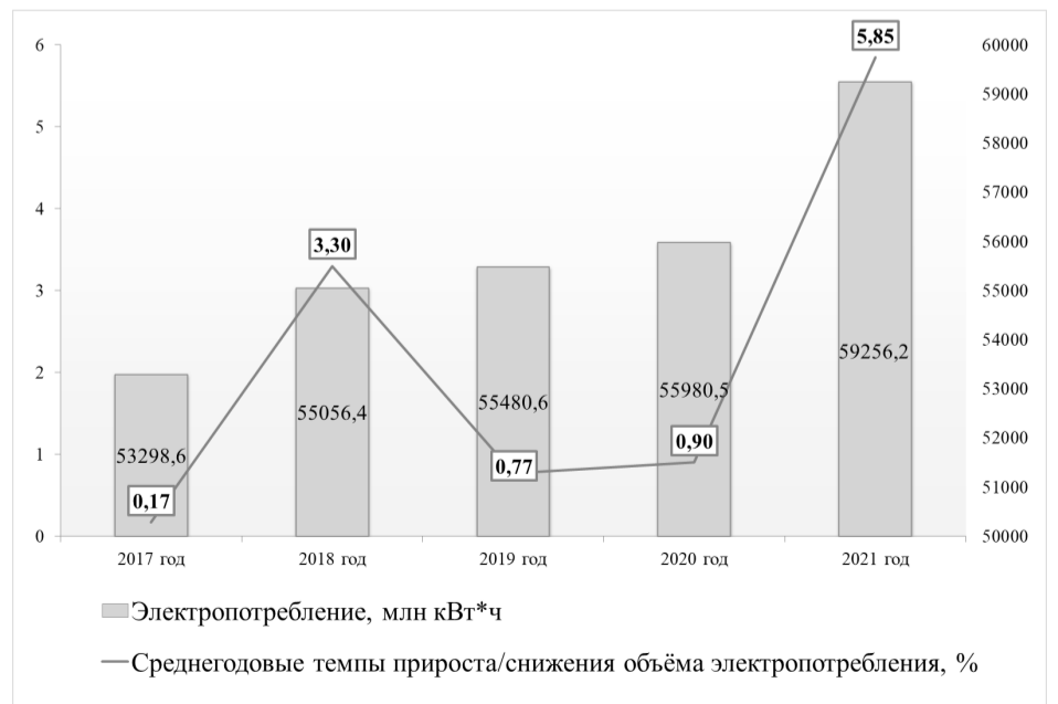
Рисунок 2.5.1. Динамика потребления электроэнергии в энергосистеме Иркутской области
