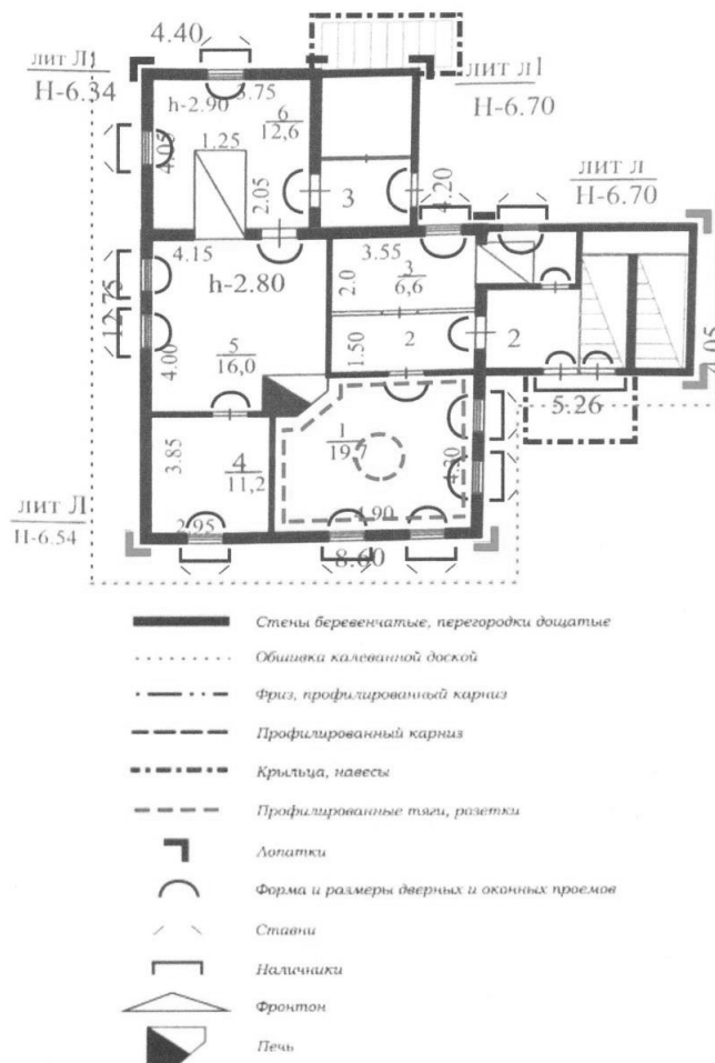
Дом лит. Л. Схема расположения предмета охраны (ценных элементов) первого этажа
