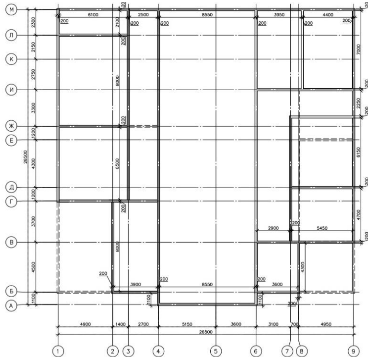
Рис. 4. Планировочная структура второго этажа.
