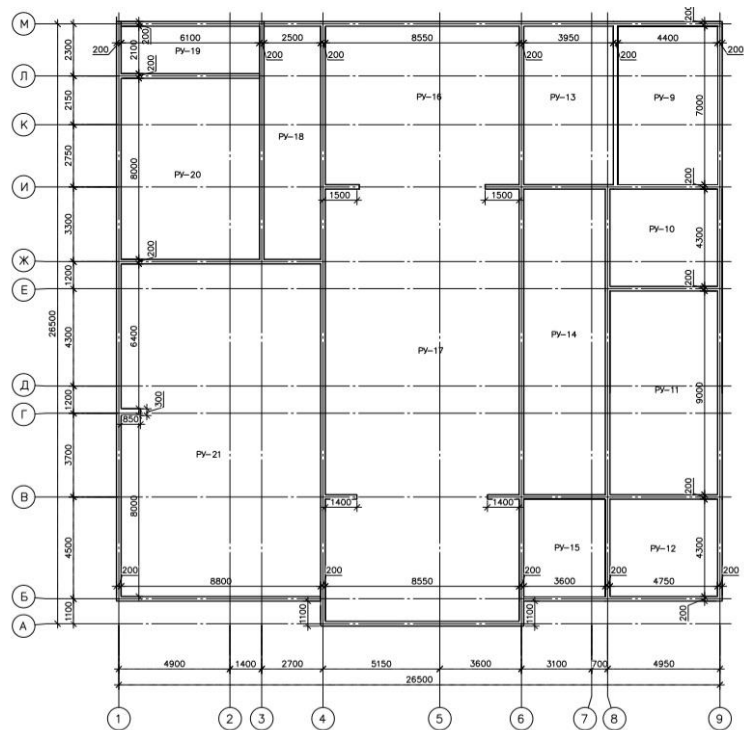
Рис. 3. Планировочная структура первого этажа.
