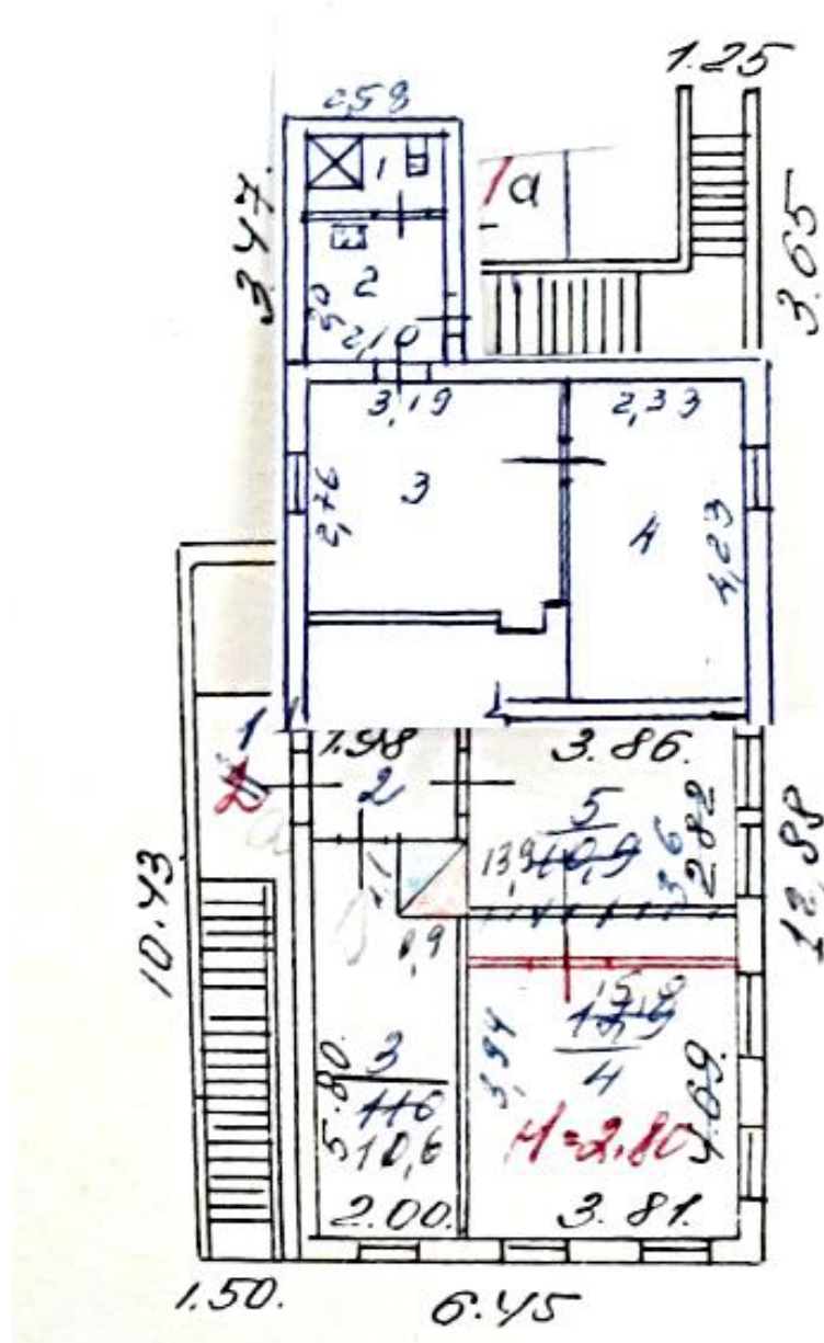
Рис. 7. План 1-го этажа. Архив БТИ, 1987 г. с изменениями 1989 г.
