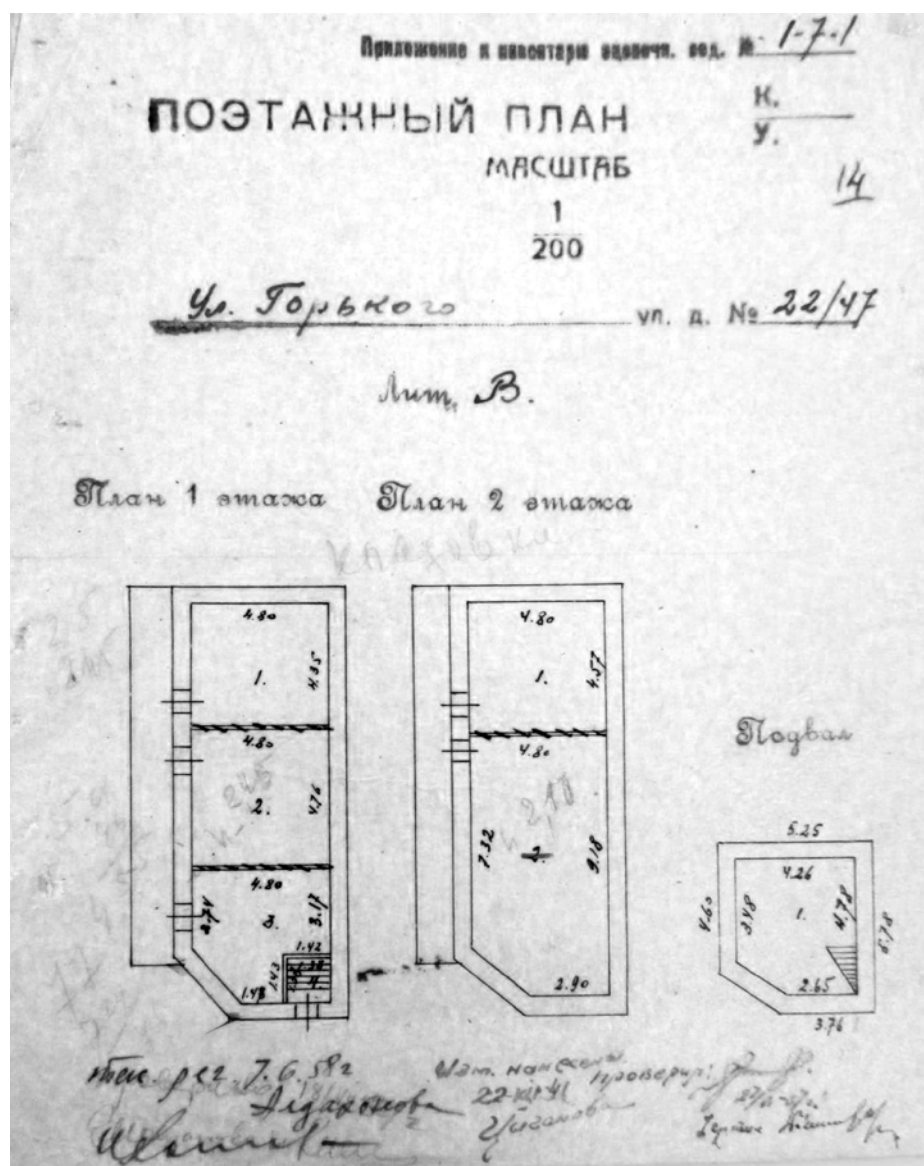
Рис. 5 - Поэтажные планы. Архив БТИ, 1937 г. с изменениями 1941 г., 1958 г.
