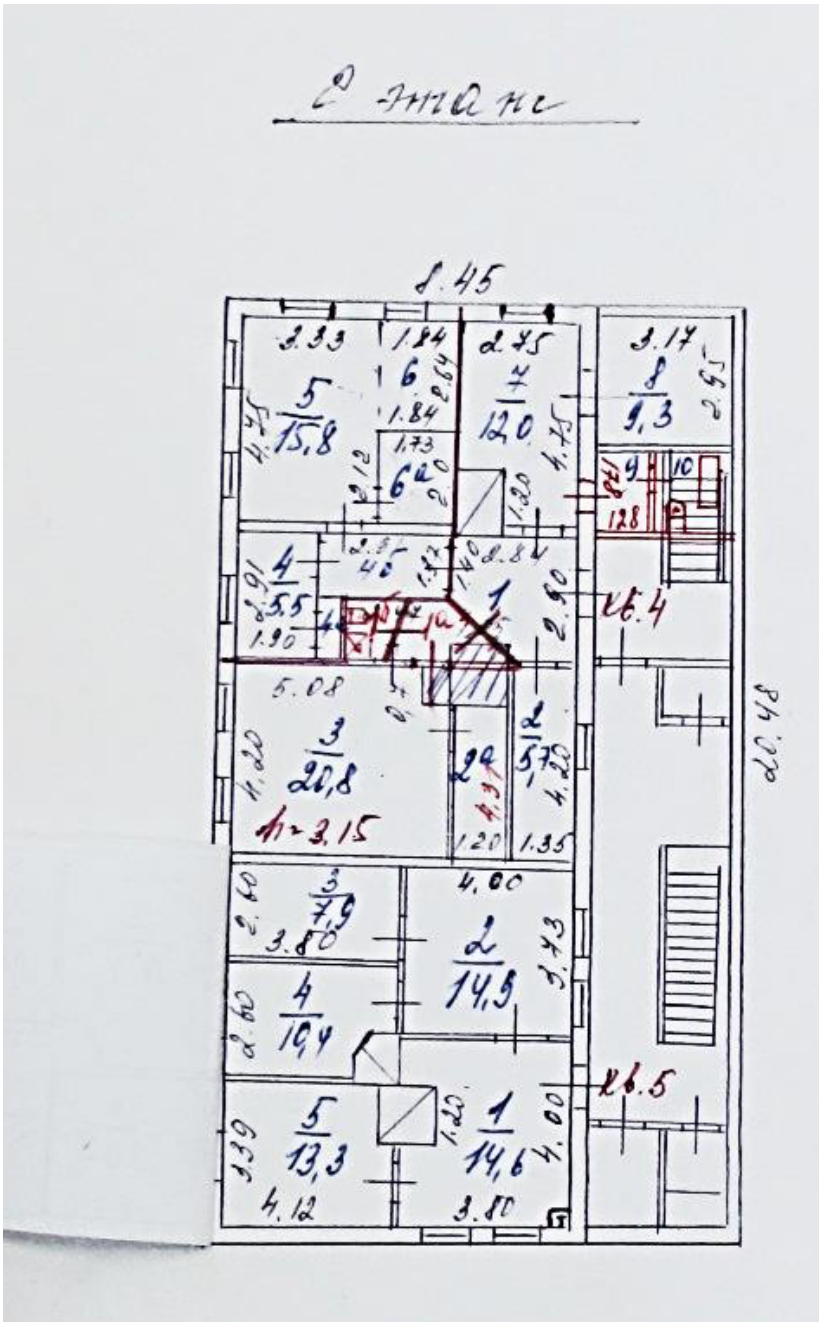
План 2-го этажа. Архив БТИ, 1998 г.
