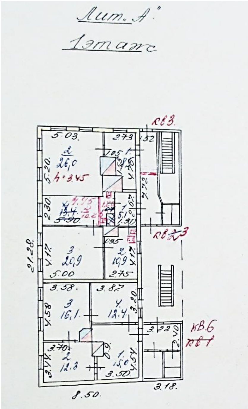
Рис. 6 - План 1-го этажа. Рис. 6 - Архив БТИ, 1987 г. с изменениями 1989 г., 1990 г.
