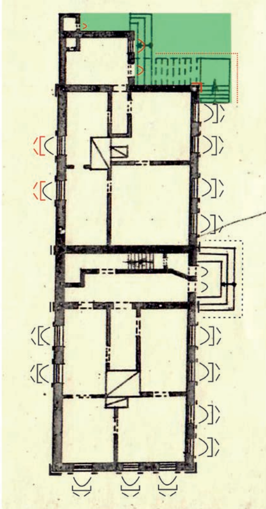
Схема расположения предмета охраны (ценных элементов) первого этажа.
