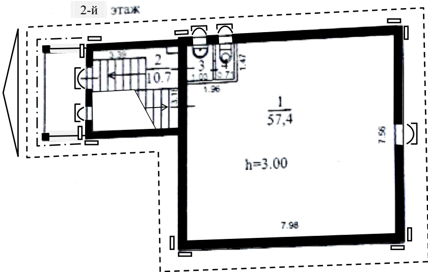
Схема расположения предмета охраны (ценных элементов) второго этажа.
