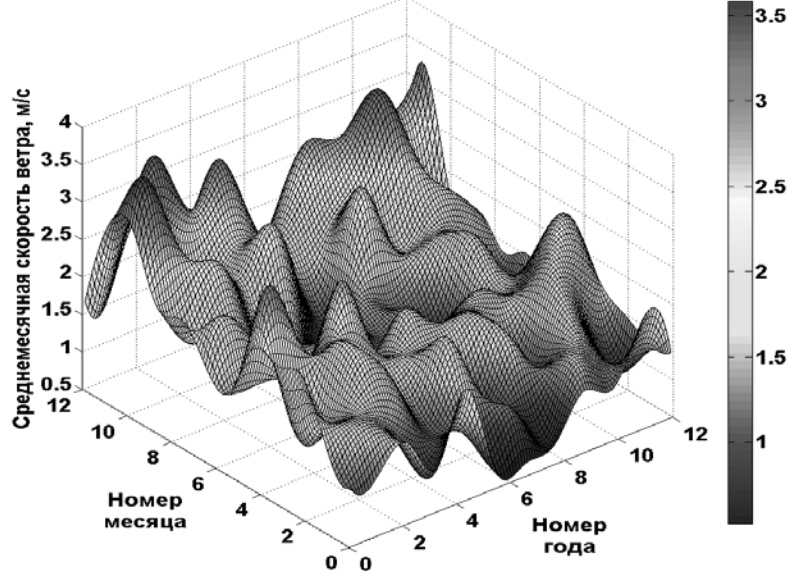
Рисунок 3.8 – График изменения среднемесячных скоростей ветра для с. Подволочное Среднегодовые значения скорости ветра не превышают 2,1 м/с, в осенние и зимние месяцы не более 1,2 м/с.
