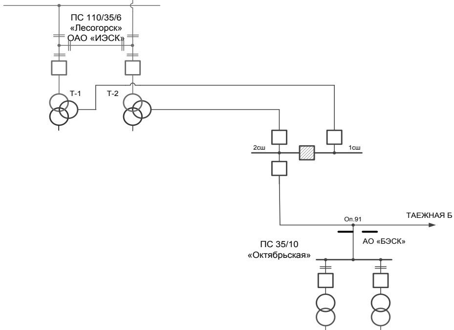
Рис. 3.2.9. Схема внешнего электроснабжения ПС 35 кВ «Октябрьская».
