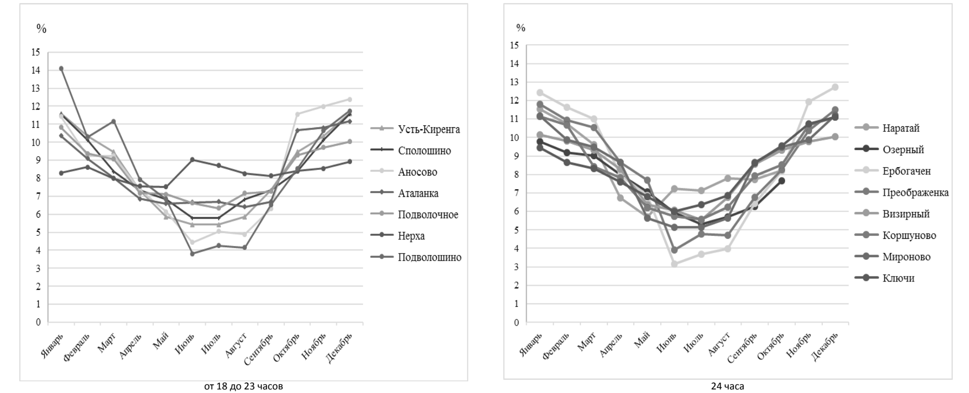
Рисунок 1.10 – Графики годового потребления электроэнергии в зависимости от числа часов работы энергоисточника
