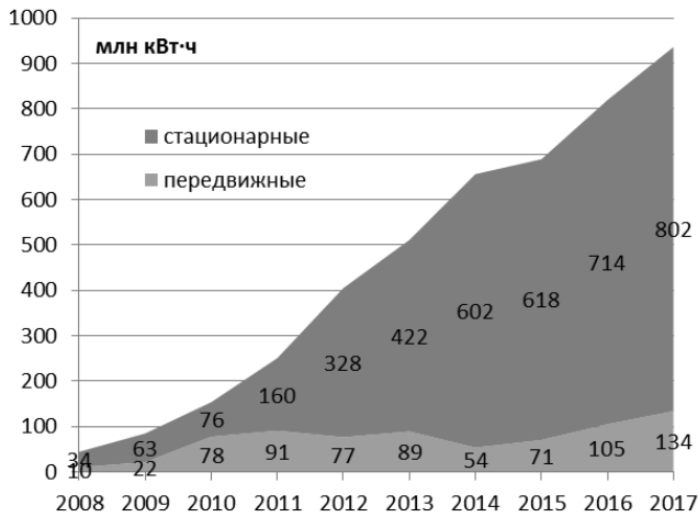
Рисунок 1.2 – Динамика выработки электроэнергии малыми электростанциями
