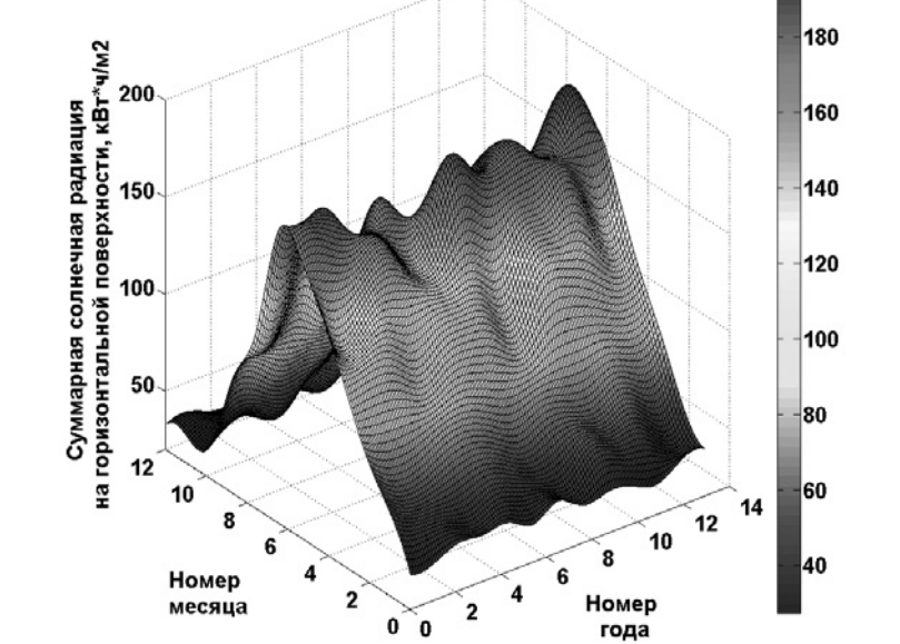
Рисунок 3.18 – График изменения суммарно солнечная радиация в с. Вершина Тугтуры
