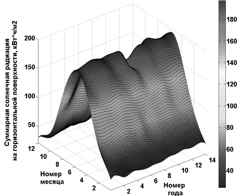
Рисунок 3.16 – График изменения суммарной солнечная радиация в д. Ключи
