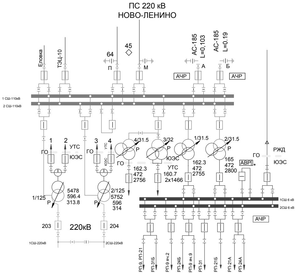
Рис. 1.1.3.5. Схема ПС 220 кВ Ново-Ленино.
