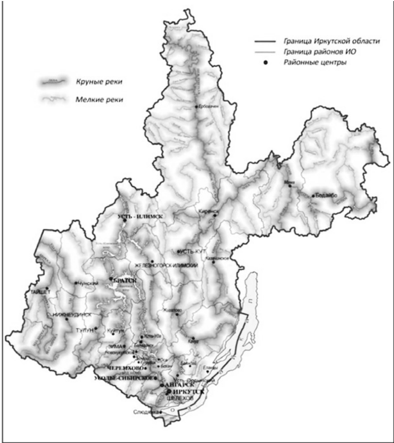
Рисунок 3.19 – Сеть водотоков на территории области
