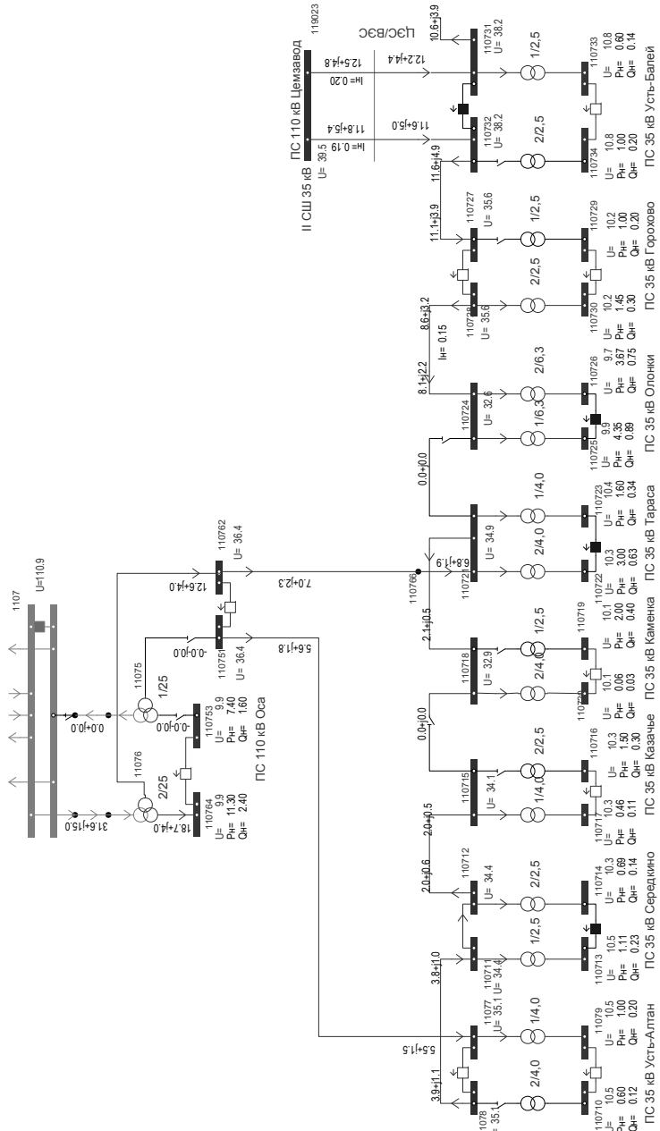
Рис. 1.1.3.3в. Ремонт Т1 на ПС 110 кВ Оса. Режим сети 35 кВ на участке
