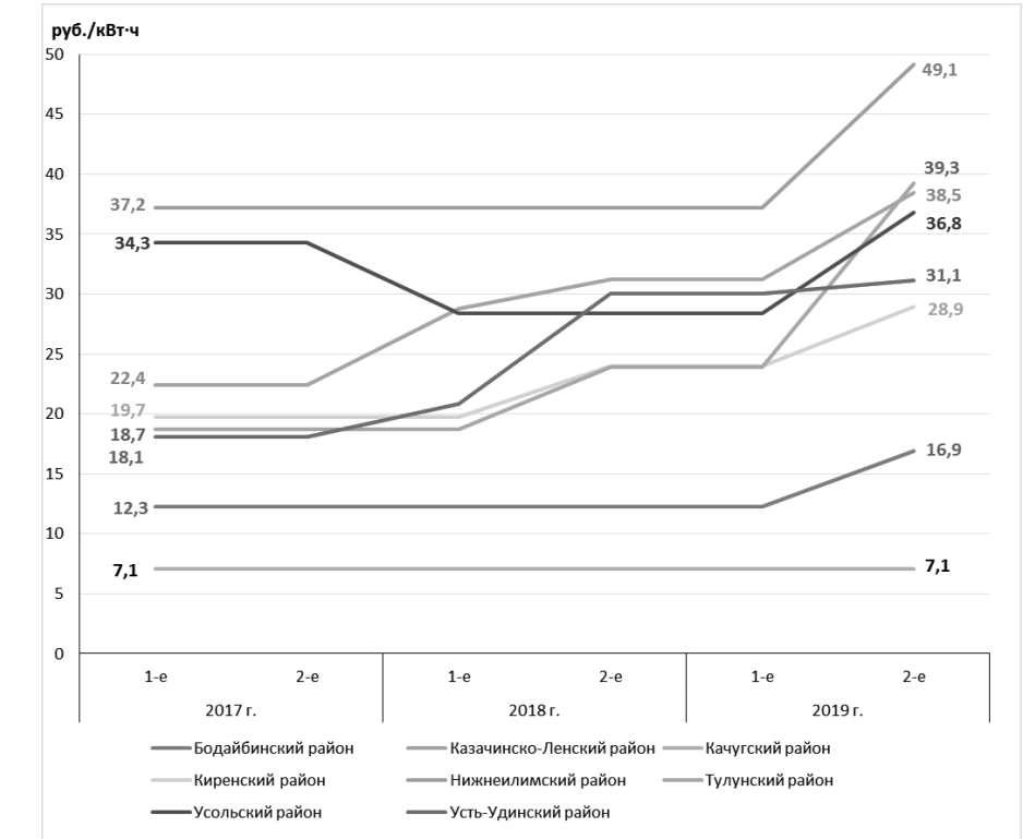
Рисунок 1.14 – Динамика экономически обоснованных тарифов на электроэнергию для децентрализованных населенных пунктов в районах с одной обслуживающей энергокомпанией
