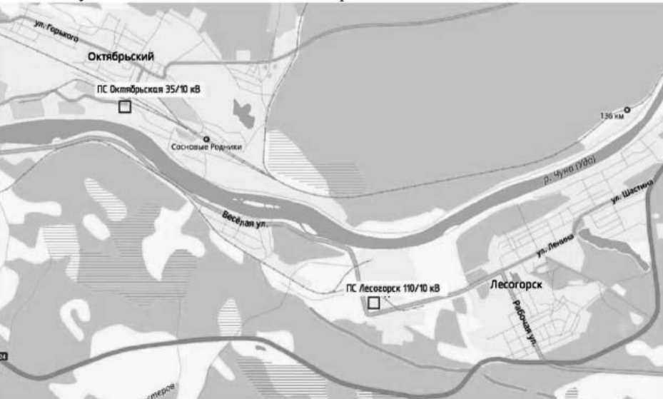
Рис. 3.2.10. Расположение ПС 35/10 кВ «Октябрьская».
