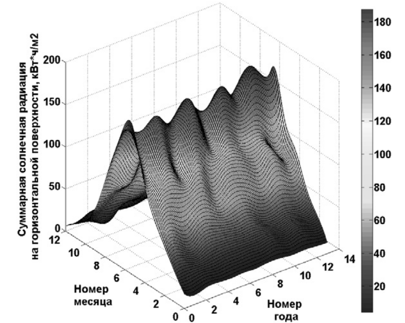
Рисунок 3.14 – График изменения суммарной солнечная радиация в с. Хамакар
