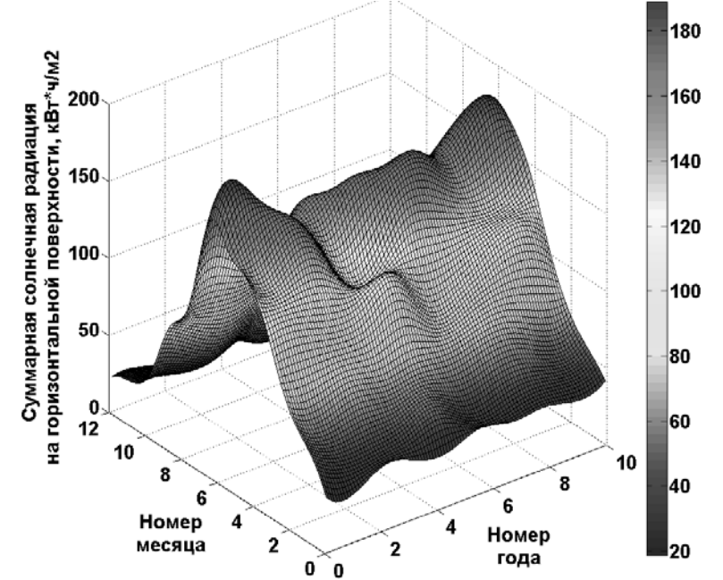
Рисунок 3.17 – График изменения суммарной солнечная радиация в с. Подволочное
