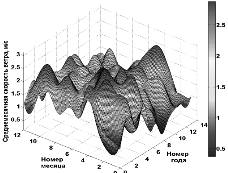
Рисунок 3.5 – График изменения среднемесячных скоростей ветра для с. Хамакар Среднегодовые значения скорости ветра не превышают 2,7 м/с, в осенние и зимние имеют значения не более 2,5 м/с.
