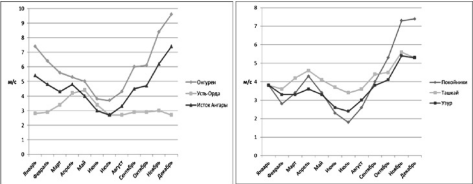
Рисунок 3.3 – Распределение в течение года среднемесячных скоростей ветра
