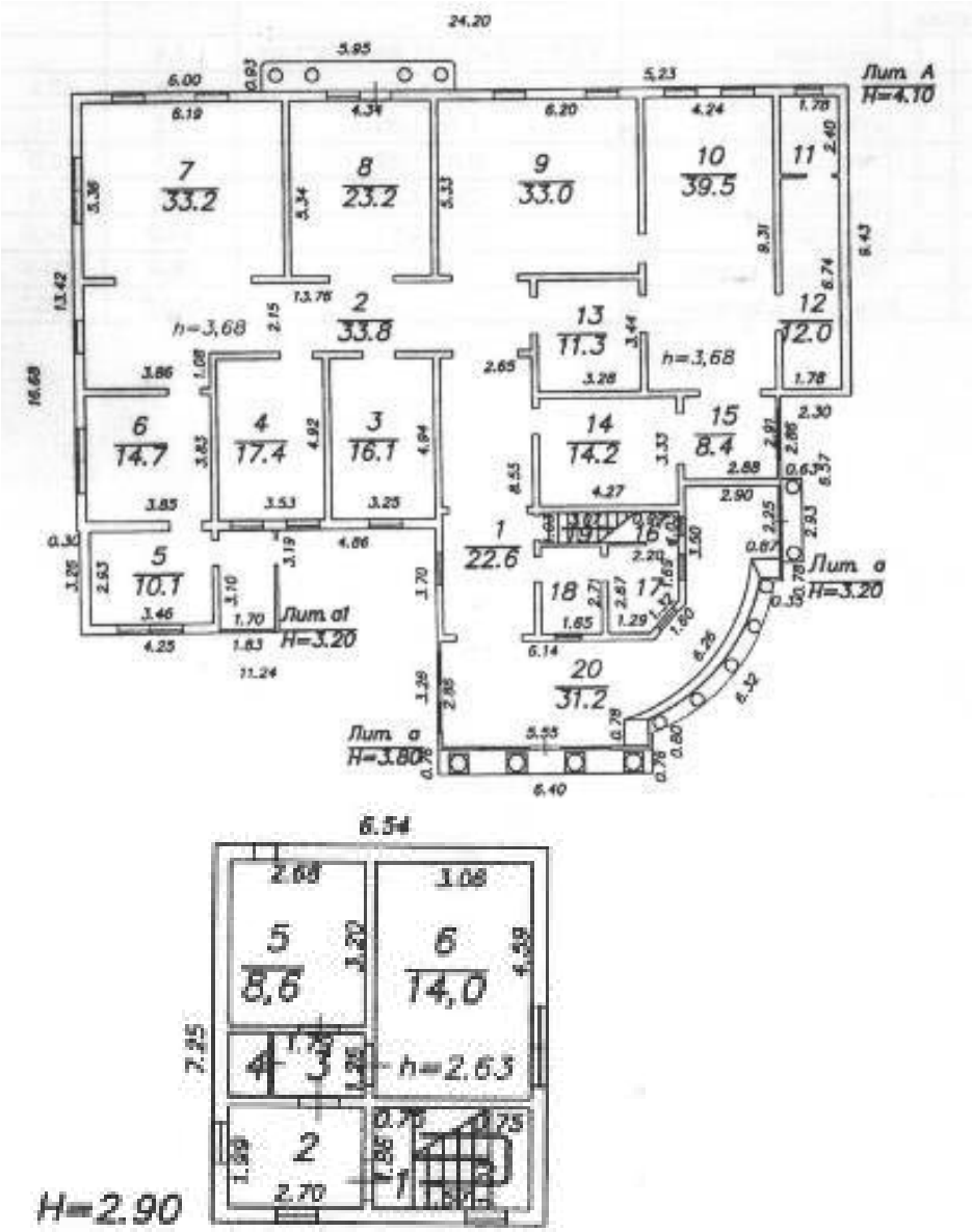
Рис. 2 - Планы 1-го 2-го этажей дома по ул. Мира, 20. (инвентаризация БТИ 2009 г.)
