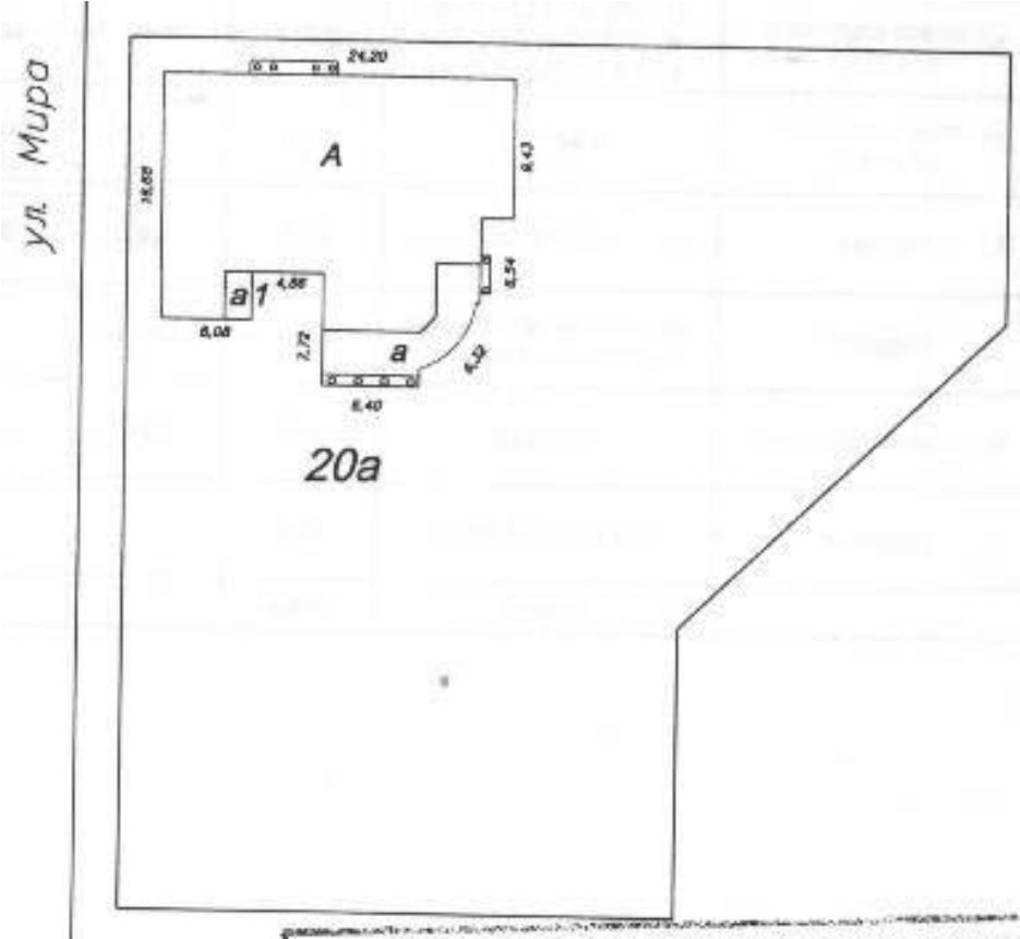
Рис. 1 - Генплан участка по ул. Мира, 20 (инвентаризация БТИ 2009 г.)
