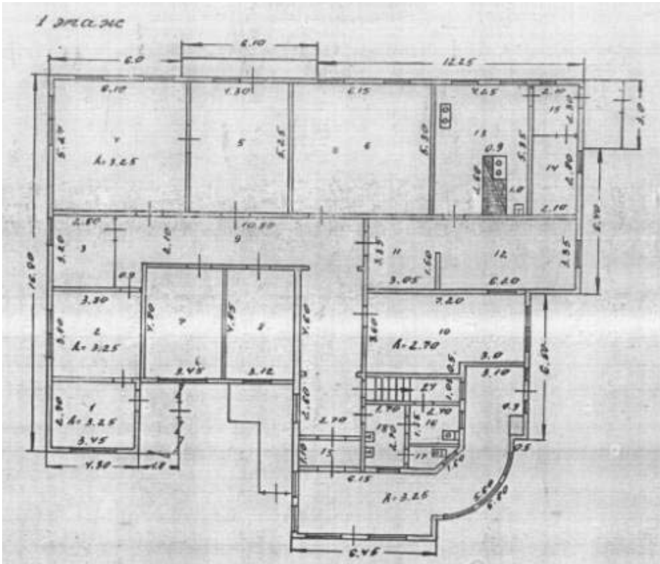
Рис. 4 - План дома. Инвентаризационные обмеры 1984 г.
