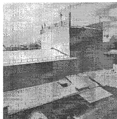
Северо-восточный фасад 3 «Театрального» корпуса – сценическая коробка и зрительный зал
