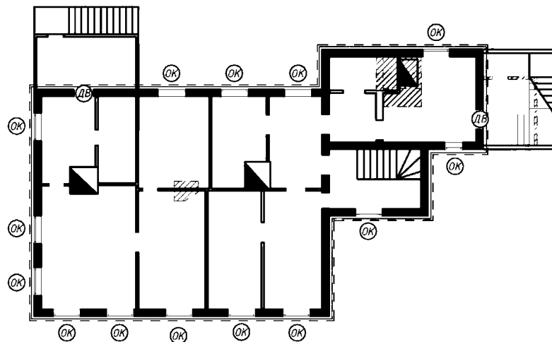
2 этаж
