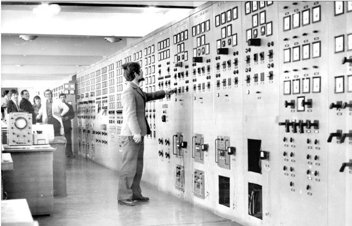
1976. С.С. Смирнов начинает эксперимент на электродинамической модели
