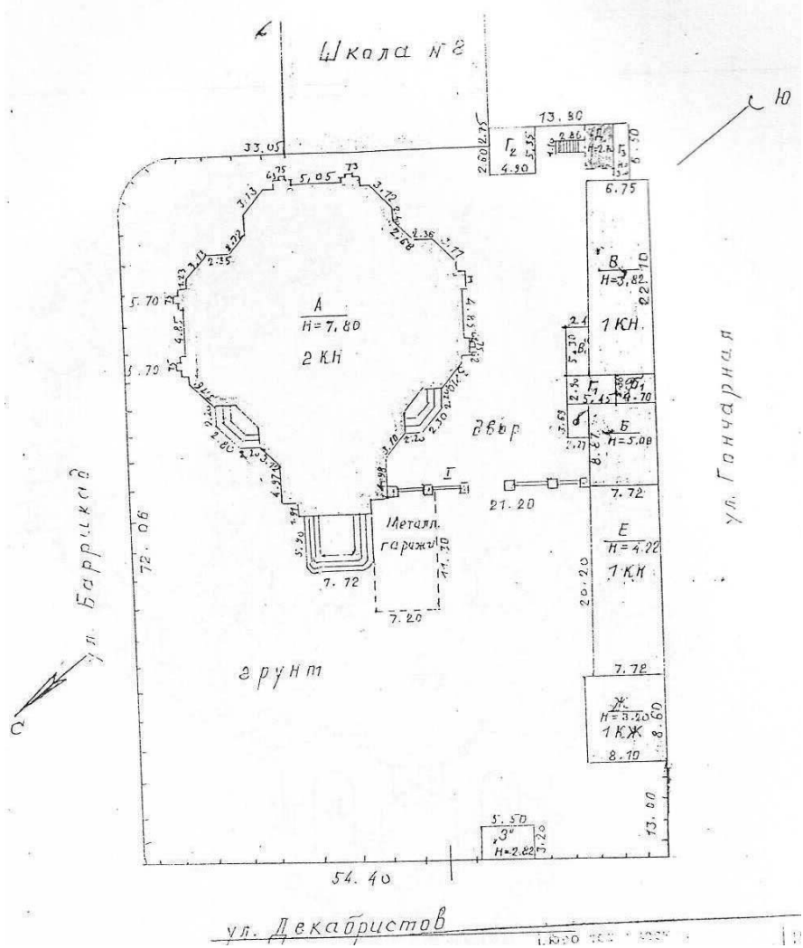
Рис. 1 - Схема генплана объекта
