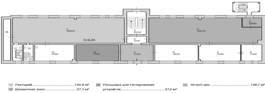
Рисунок 4. Зонирование 4 этажа детского технопарка «Кванториум Байкал»
